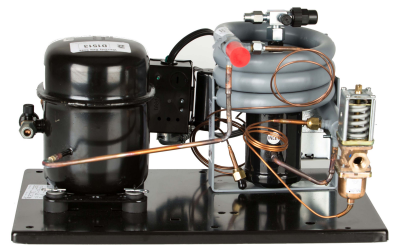
(1) Condensing Unit
