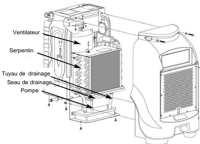
Dessin 1 DrizAir 1200
